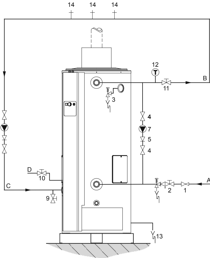
Esquema de ligação
