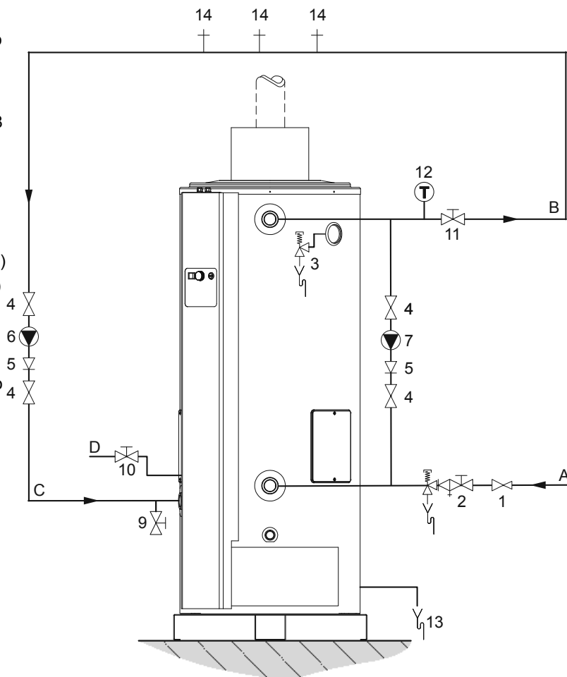
Esquema de ligação
